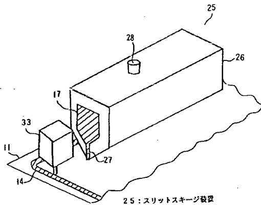
25 : スリットスキージ装置
